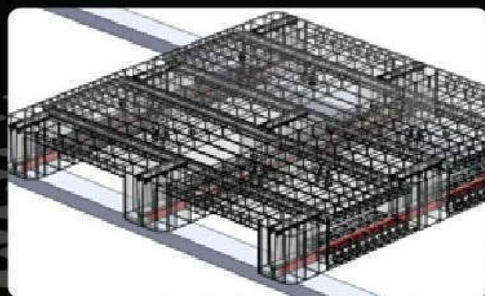
แนวเหล็กยาว เพื่อรับน้ำหนักขณะยกขึ้น Rack
