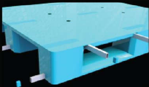
ตำแหน่งใส่เหล็ก เพิ่มความแข็งแรง
